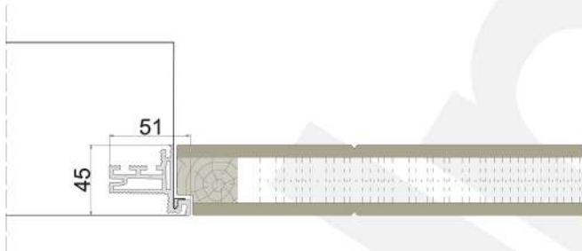
SISTEMA KO-ZERO - RASO PARETE
