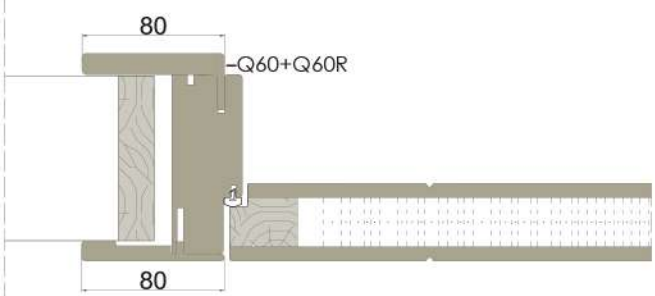
SISTEMA B-DUE - FILO MURO TIRARE
