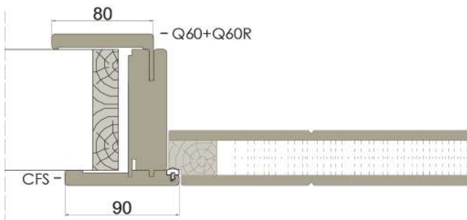
SISTEMA B-DUE - FILO MURO TIRARE
